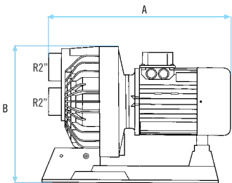
Bomba monofásica (Cód. 11505) Singlephase pump (Code 11505) Potencia 1,50 kW. Monofásica 230 V 50 Hz Power 1,50 kW. Singlephase 230 V 50 Hz
