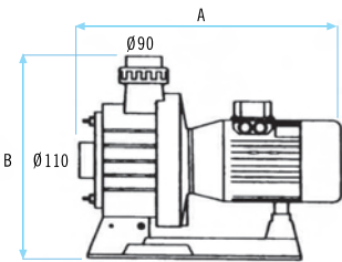
Bomba trifásica (Cód. 11509) Three-phase pump (Code 11509) Potencia 3,30 kW. Trifásica 230/400 V 50 Hz Power 3,30 kW. Three-phase 230/400 V 50 Hz
