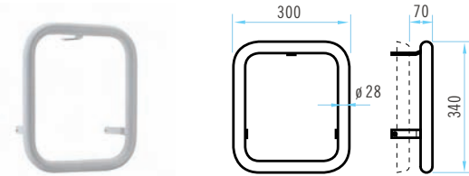
Rectangular en inox. AISI-316 pintado (Cod. 09447) S.S. AISI-316 square painted (Cod. 09447)
